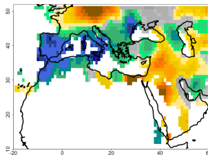
Drier Prob. %
